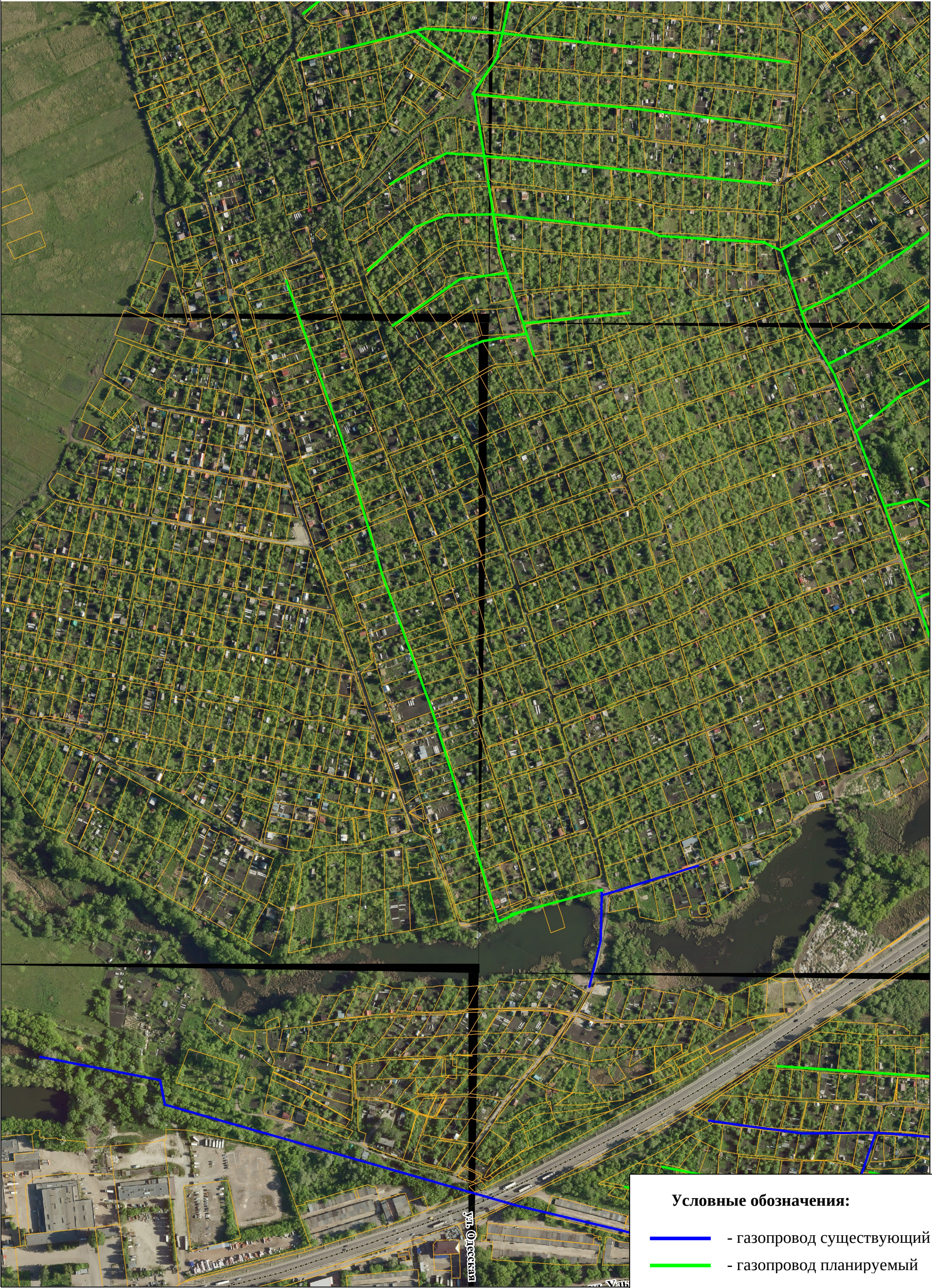
Схема планируемых объектов газоснабжения города Пензы (СНТ 40 лет ВЧК)
