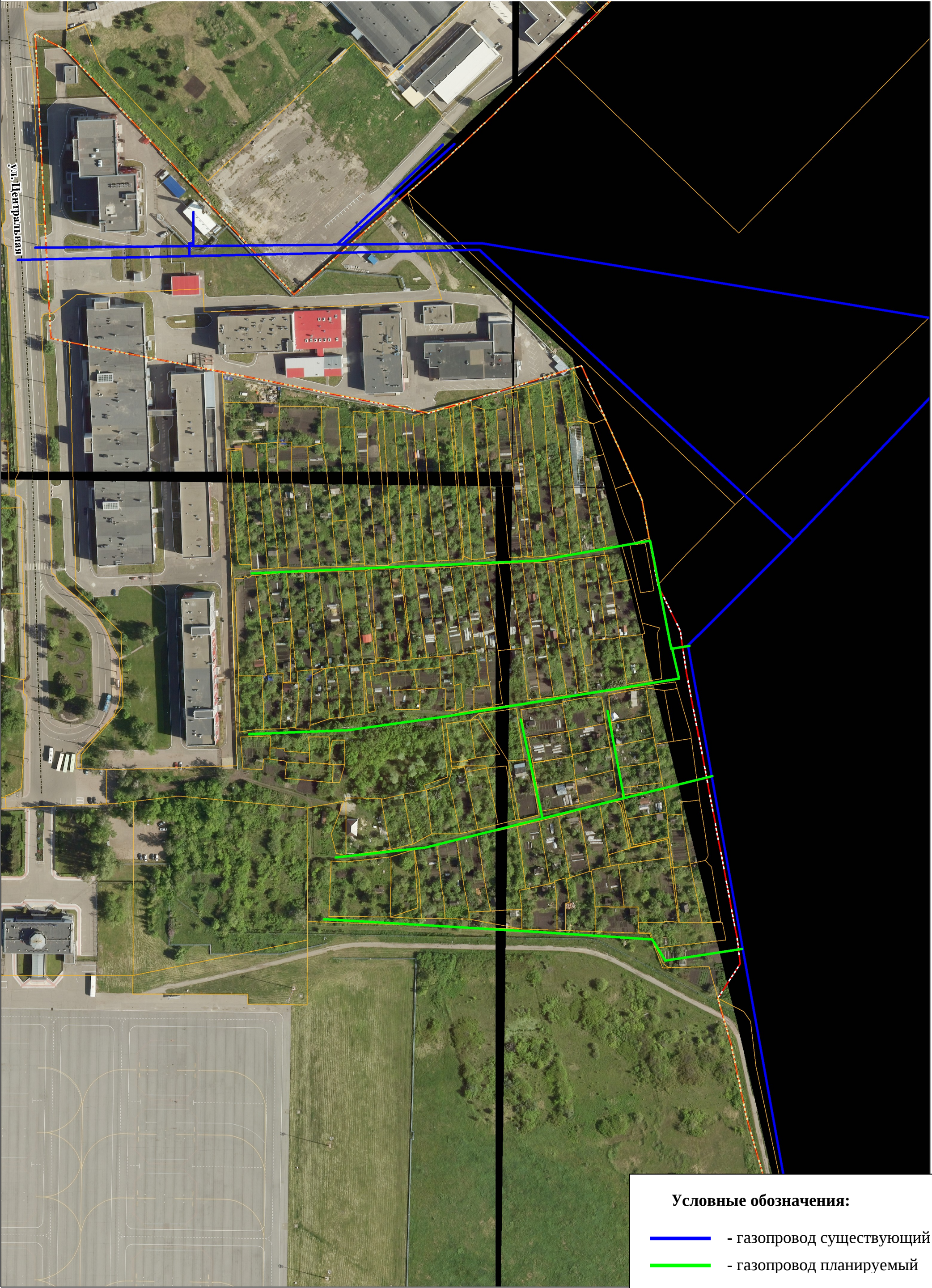
Схема планируемых объектов газоснабжения города Пензы (СНТ Авиатор-1, С/Т Авиатор-2)
