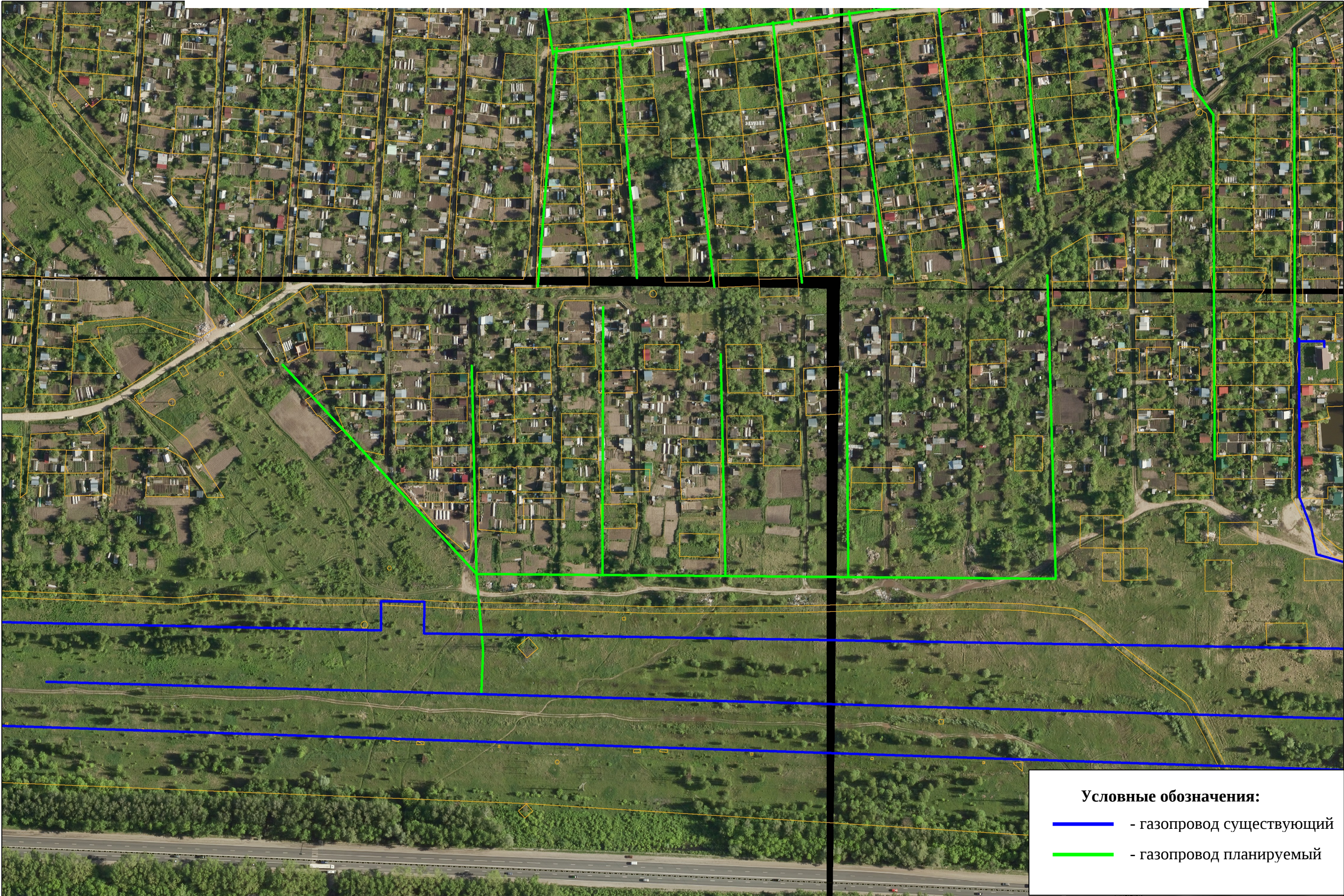
Схема планируемых объектов газоснабжения города Пензы (СНТ Виктория)
