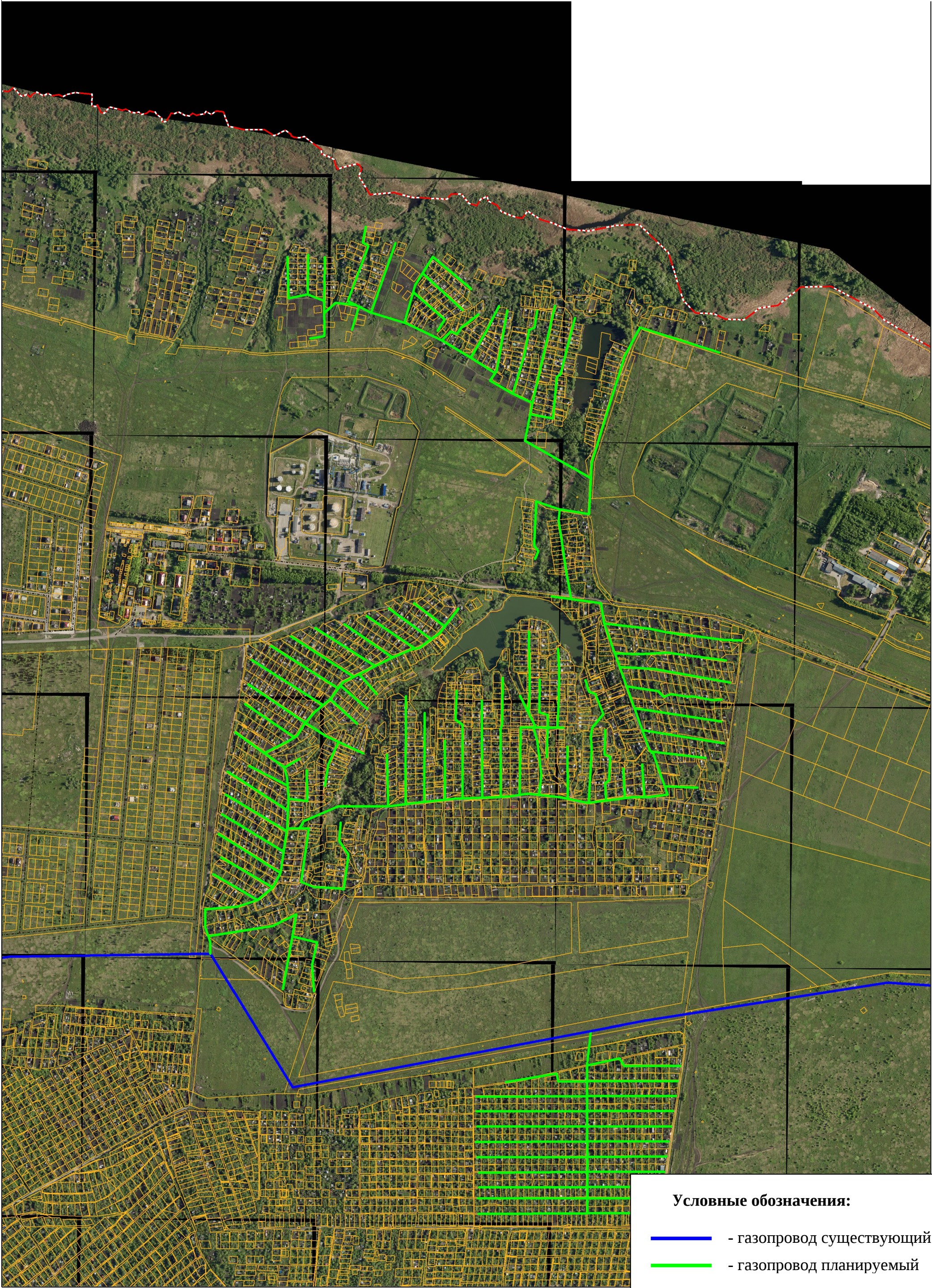
Схема планируемых объектов газоснабжения города Пензы (СНТ Гудок)
