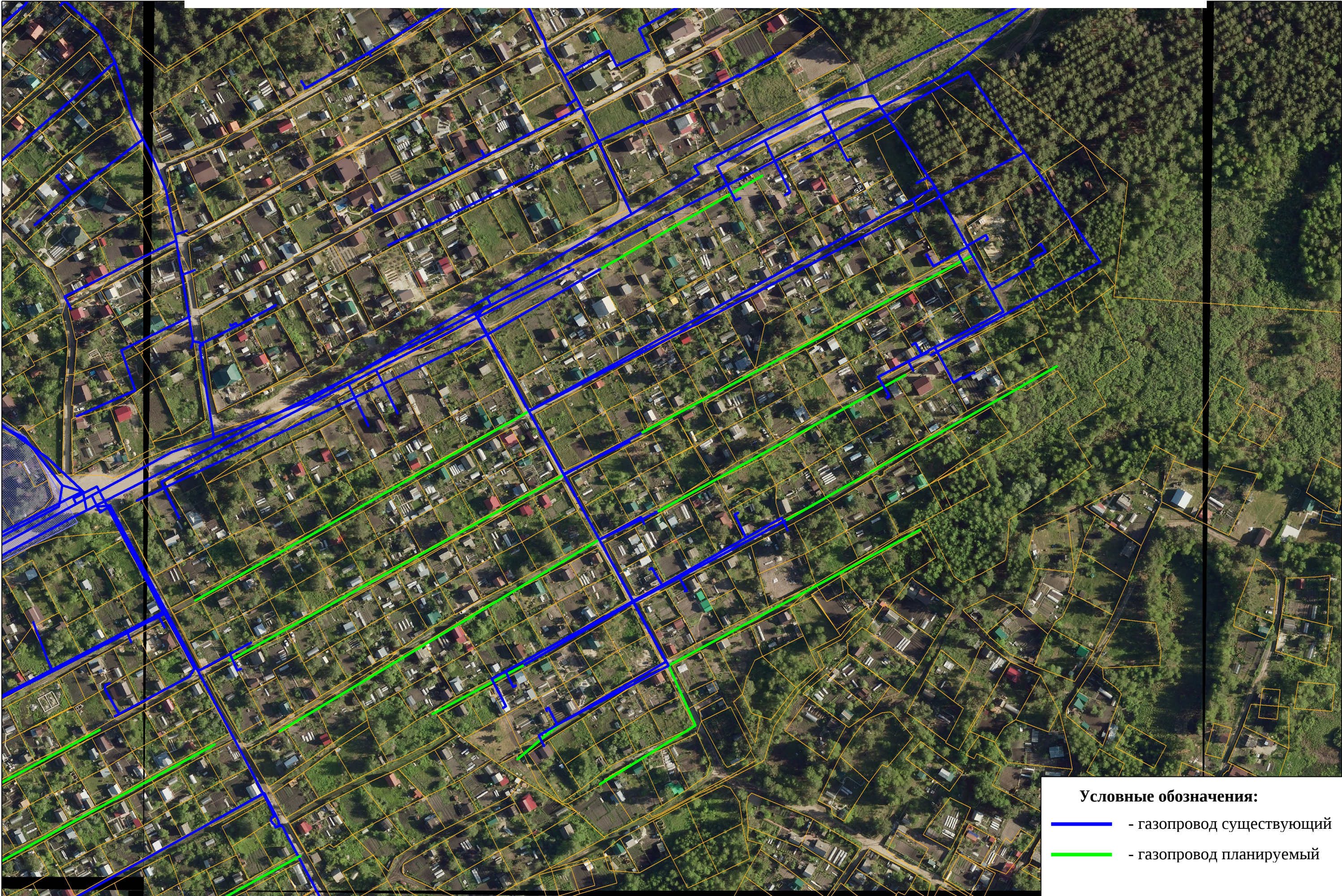
Схема планируемых объектов газоснабжения города Пензы (СНТ Дизелист)
