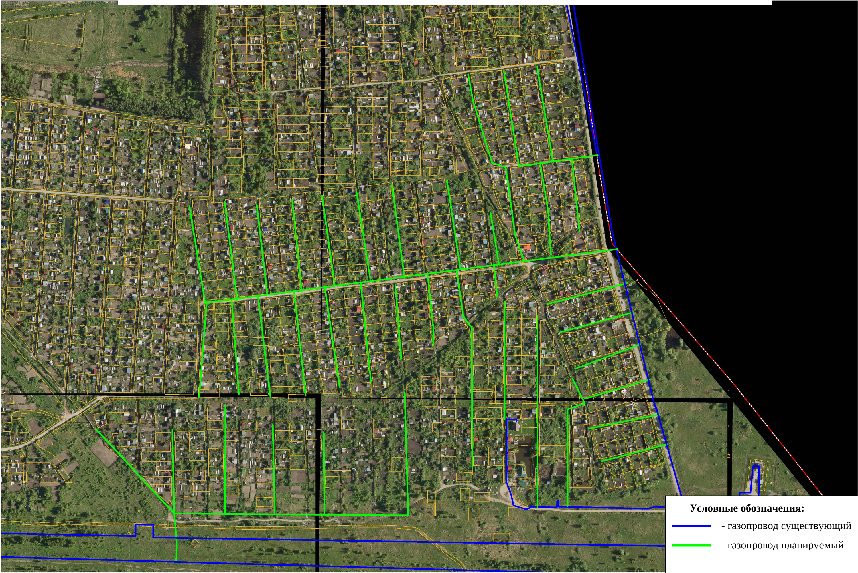
Схема планируемых объектов газоснабжения города Пензы (СНТ Здоровье, СНТ Сигнал)
