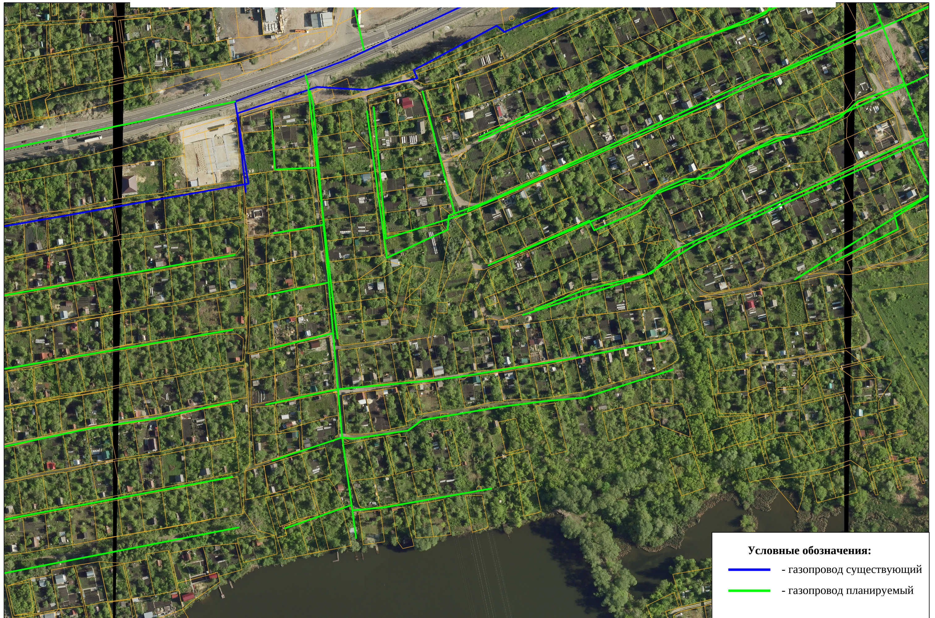
Схема планируемых объектов газоснабжения города Пензы (ТСН Механизатор)
