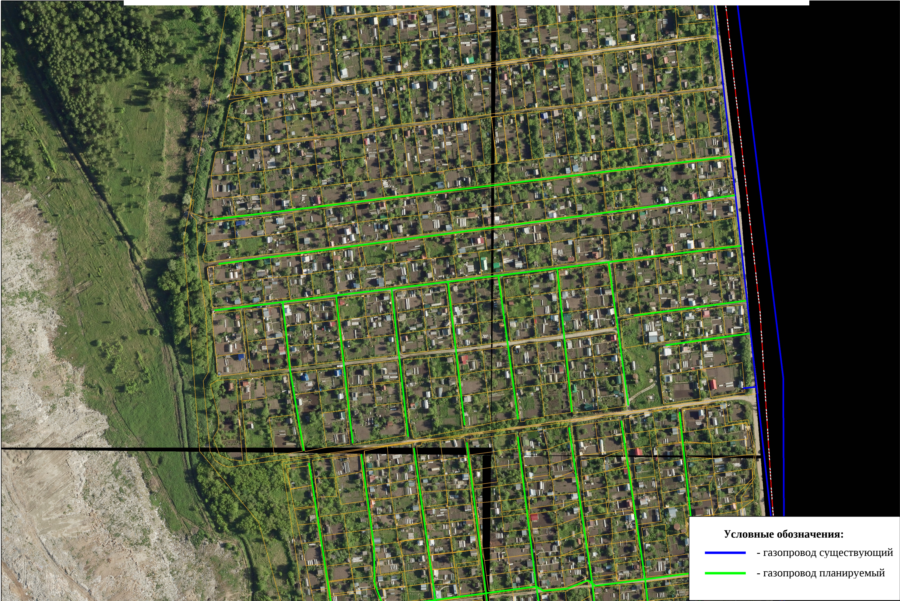
Схема планируемых объектов газоснабжения города Пензы (СНТ Пчелка)
