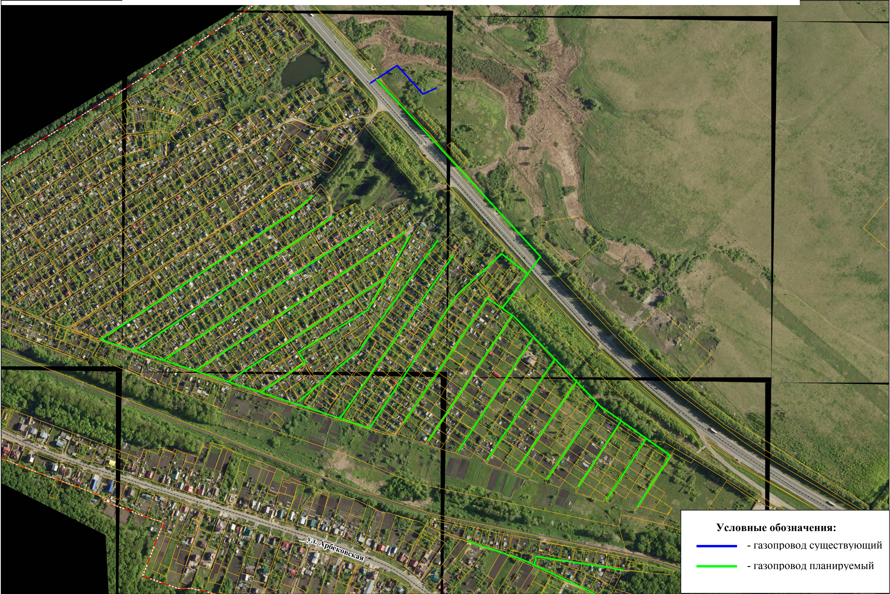
Схема планируемых объектов газоснабжения города Пензы (СНТ Ромашка, СНТ Солнечное (Октябрьский район))
