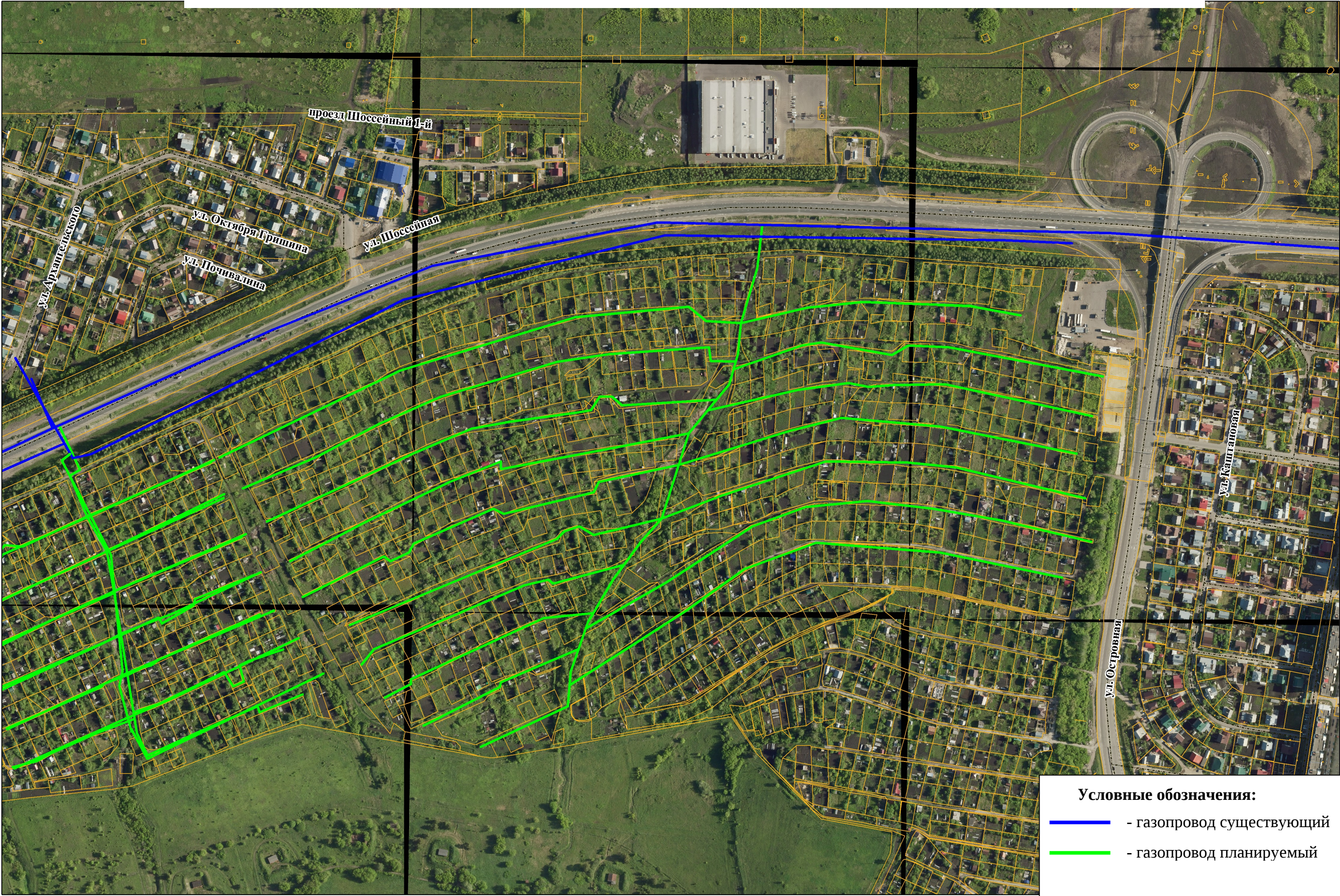
Схема планируемых объектов газоснабжения города Пензы (СНТ Север)
