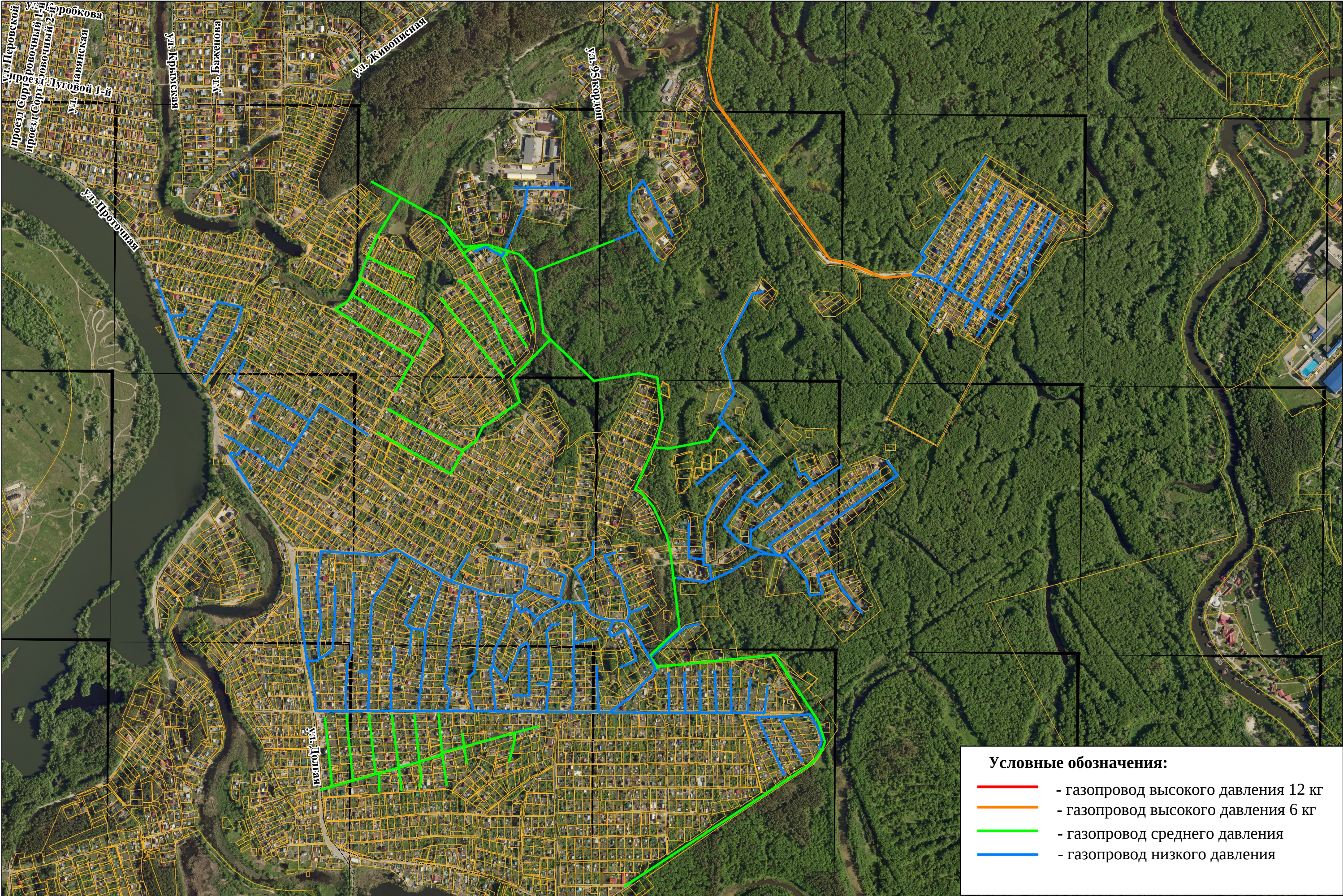
Схема планируемых объектов газоснабжения города Пензы (СНТ Весна-1, СНТ Дружба-2, СТ Коммунальник, СНТ Озерное, СНТ Энергетик-2, СНТ Весна (службы быта Облпромсовета), СНТ Дружба (Барковка))
