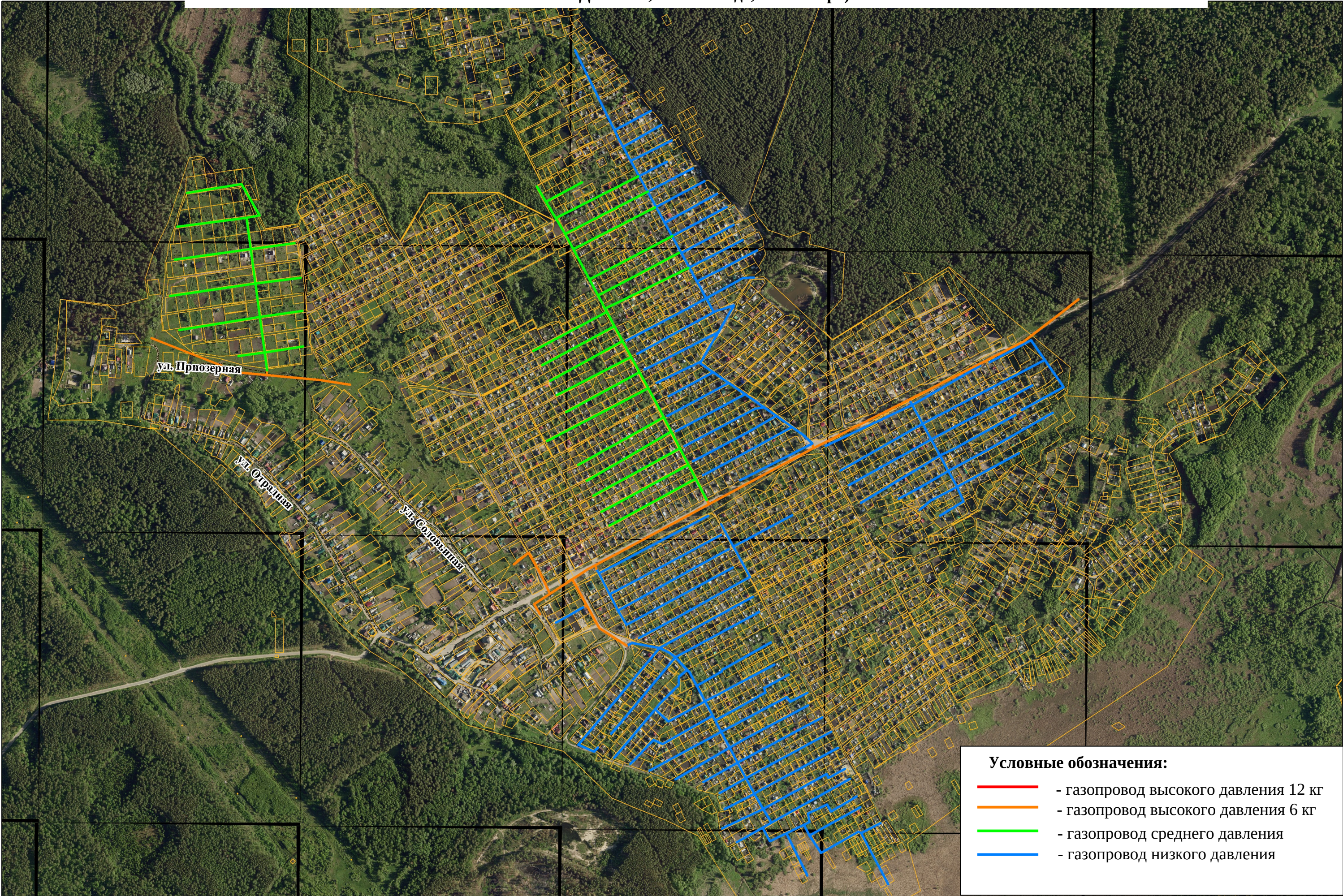
Схема планируемых объектов газоснабжения города Пензы (СНТ Знание, СНТ Романтики, СНТ Машиностроитель, СНТ Бодрость, СНТ Дизелист, СНТ Победа, СНТ Астра)
